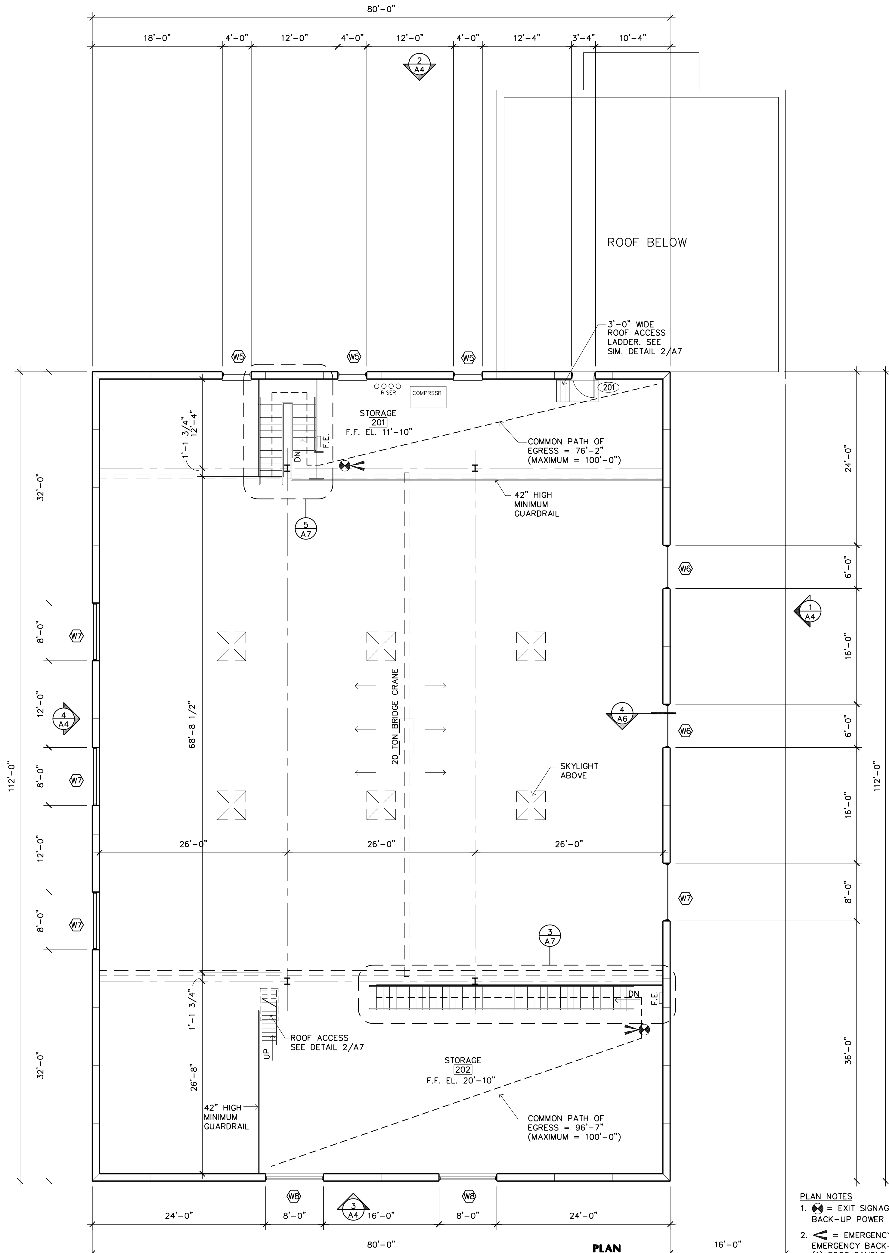
2 MEZZANINE PLAN A2 SCALE: 1/8" = 1'-0"
